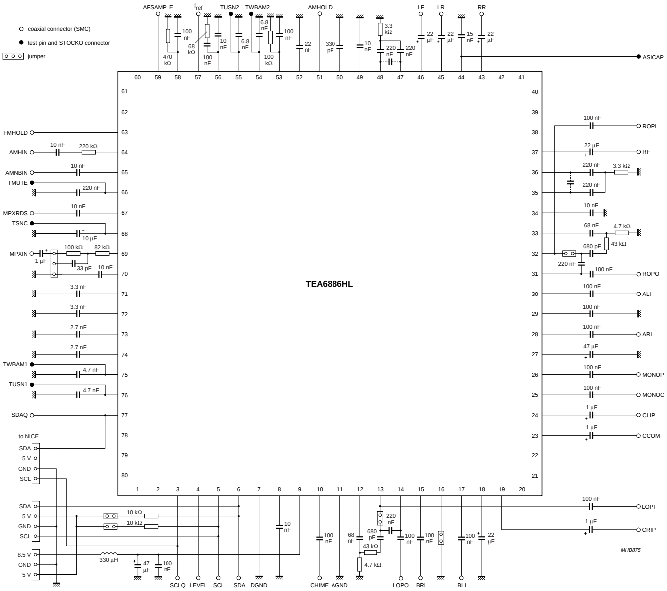
Fig.21 Test circuit.
